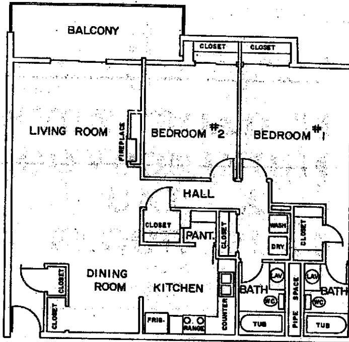
UNIT 'B'
